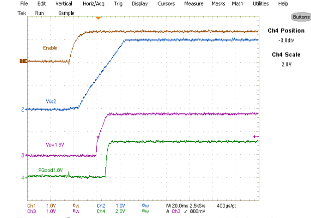
Fig.15: Start-up sequence into 20A load. Ch 1 : Enable, Ch 2 : V ss1 , Ch 3 : V o1 (2V5), Ch 4 : PGood(2V5) Fig.16: Start-up sequence into 20A load. Ch 1 : Enable, Ch 2 : V ss2 , Ch 3 : V o2 (1V8), Ch 4 : PGood(1V8)
